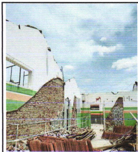
FOTO 11- DEMOLIÇÃO DE ALVENARIA DE BLOCO FURADO, DE FORMA MANUAL, SEM REAPROVEITAMENTO.
