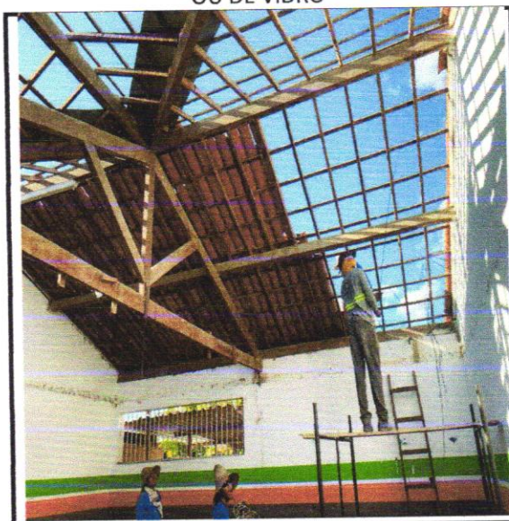
FOTO - 04: DEMOLICAO DE TELHAS CERAMICAS OU DE VIDRO
