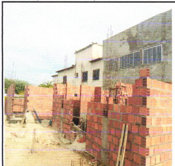
FOTO - 06 ALVENARIA DE VEDAÇÃO DE BLOCOS CERÂMICOS FURADOS NA HORIZONTAL DE 9X19X19 CM (ESPESSURA 9 CM) E ARGAMASSA DE
