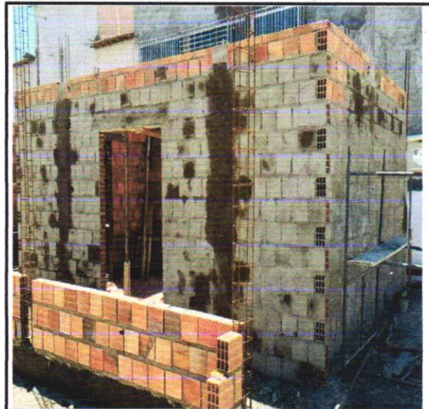
FOTO - 08 CHAPISCO APLICADO EM ALVENARIAS E ESTRUTURAS DE CONCRETO INTERNAS, COM COLHER
