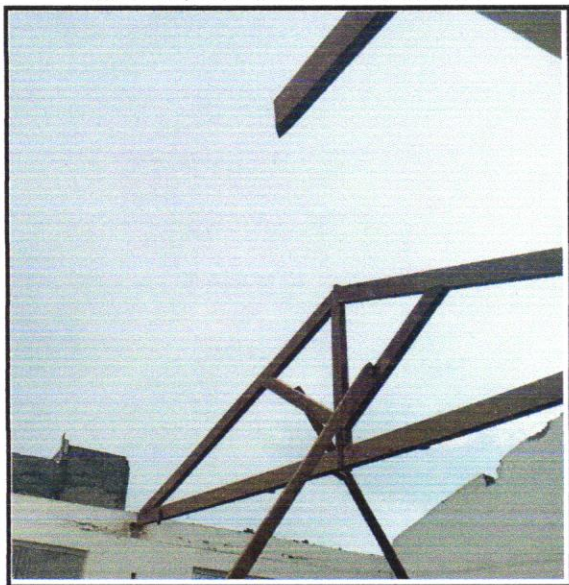
FOTO 15- REMOÇÃO DE TESOURAS DE MADEIRA, COM VÃO MAIOR OU IGUAL A 8M, DE FORMA MANUAL, SEM REAPROVEITAMENTO
