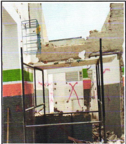
FOTO 28 - DEMOLIÇÃO DE ALVENARIA DE BLOCO FURADO, DE FORMA MANUAL, SEM
