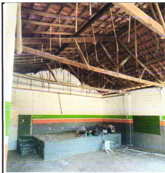
FOTO- 12 REMOÇÃO DE TESOURAS DE MADEIRA, COM VÃO MAIOR OU IGUAL A 8M, DE FORMA MANUAL, SEM REAPROVEITAMENTO
