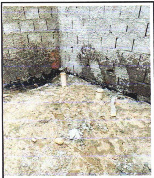
FOTO 19- CHAPISCO APLICADO EM ALVENARIAS E ESTRUTURAS DE CONCRETO INTERNAS, COM COLHER DE PEDREIRO
